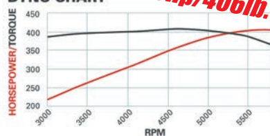
DYNO CHART
